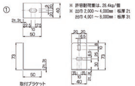
取付ブラケット
