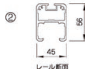
レール断面
