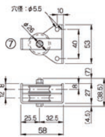
レール取付滑車 (滑車型のみ)
